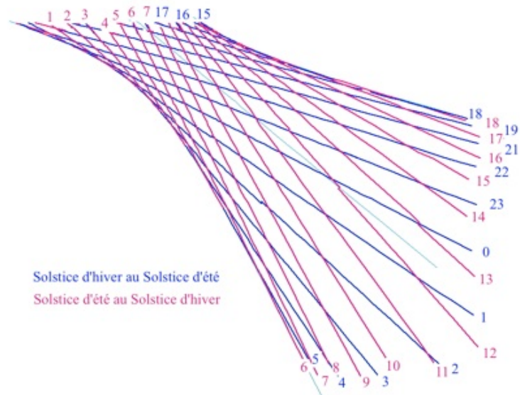
Fig.3 : Exemple de cadran « virtuel » : le cadran à heures sidérales
